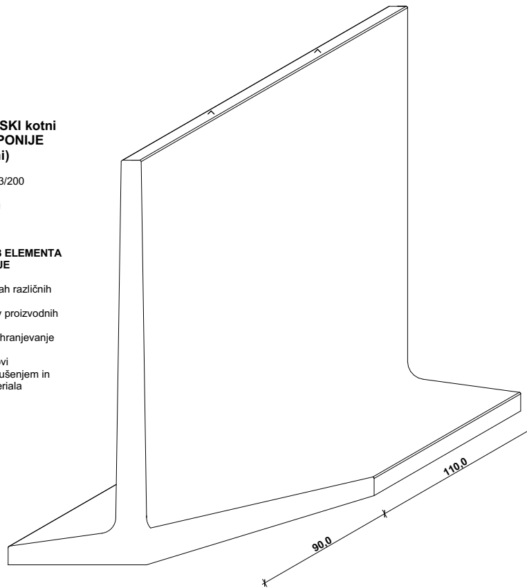
POGLED
